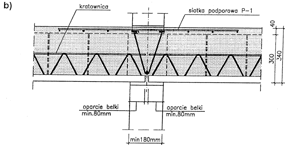
Z5-6. Zasady układania siatek płaskich a) na ścianach zewnętrznych konstrukcyjnych (i przy dylatacji), b) na ścianach wewnętrznych konstrukcyjnych
