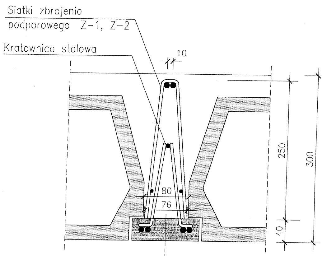
przekrój poprzeczny przez żebro w strefie podporowej
